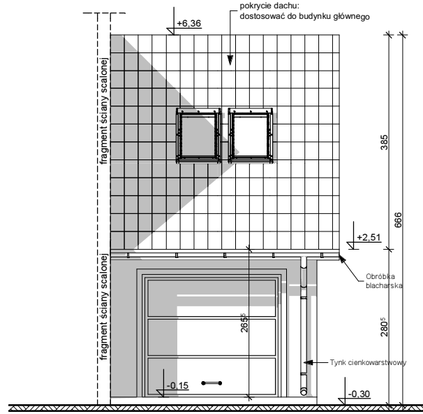
ELEWACJA FRONTOWA
