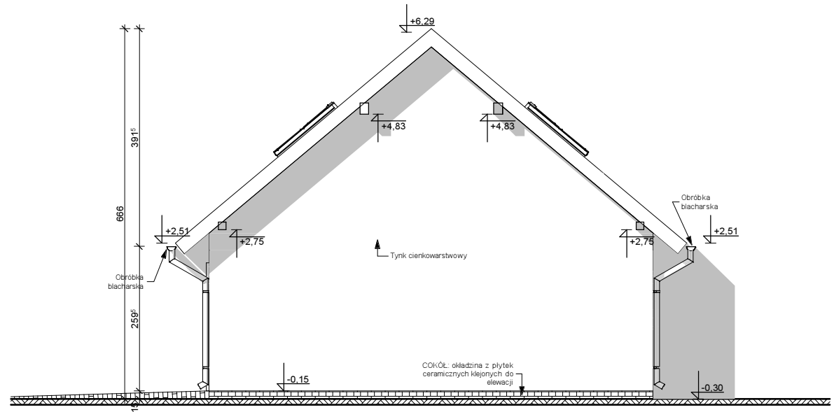
ELEWACJA BOCZNA
