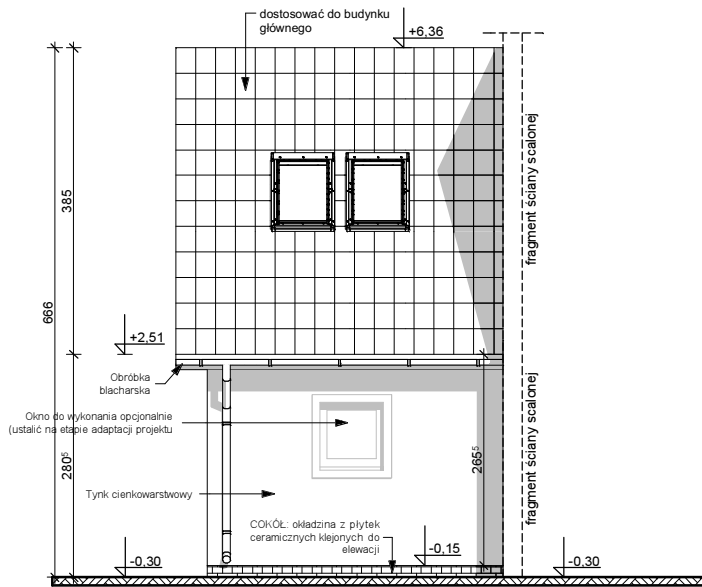
ELEWACJA OGRODOWA
